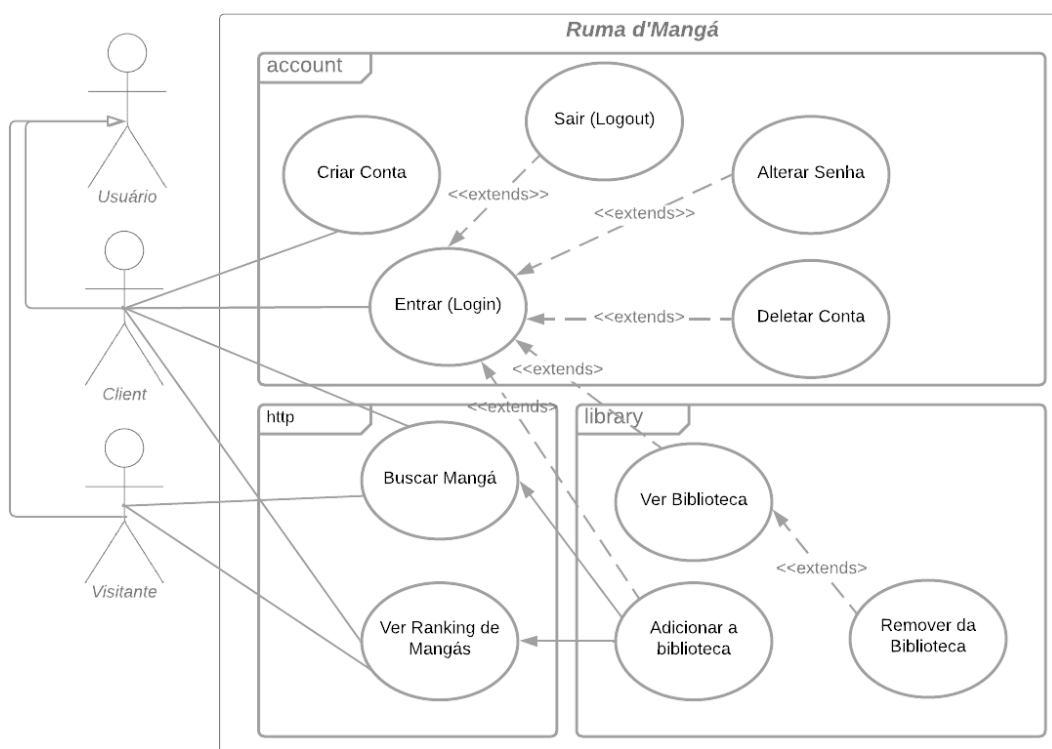
Figura 1 – Diagrama de Casos de Uso (Sistema de busca de mangá)
