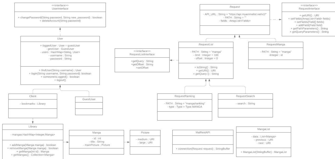
Figura 5 – Diagrama de Classe (Sistema Ruma d'Mangá)
