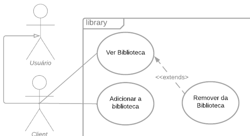
Figura 4 – Diagrama de Caso de Uso (Pacote – library)
